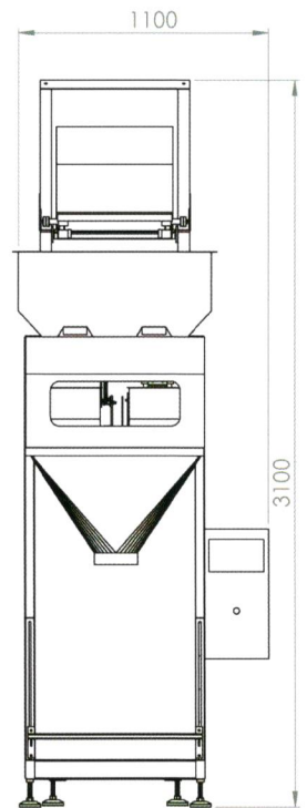
مخطط أبعاد آلة SA-12 (mm)
